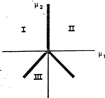
Fig. 1. T=0 .
